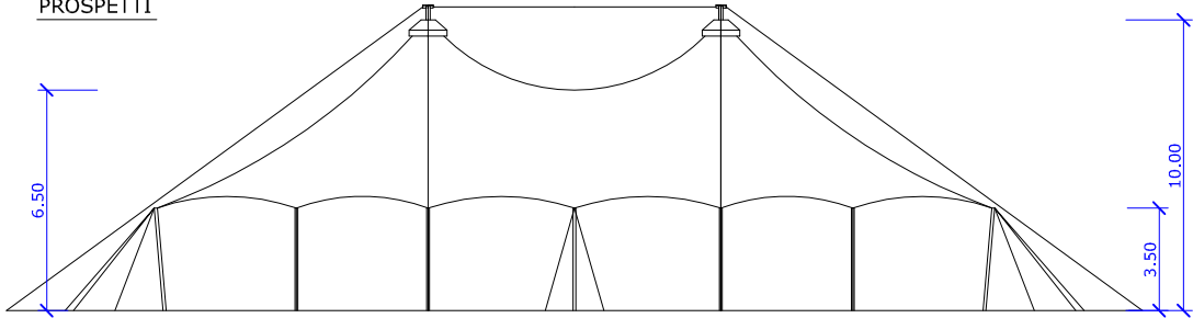
PROSPETTI
